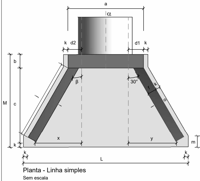
Planta - Linha simples
