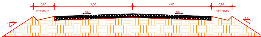
SEÇÃO TIPO DE PAVIMENTAÇÃO CORTE EIXO DE LOCAÇÃO
