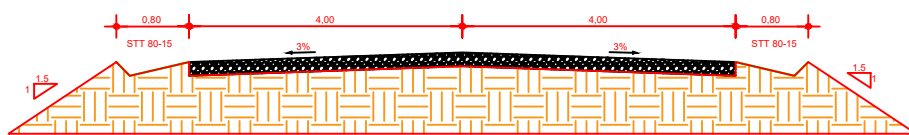
SEÇÃO TIPO DE PAVIMENTAÇÃO ATERRO EIXO DE LOCAÇÃO
