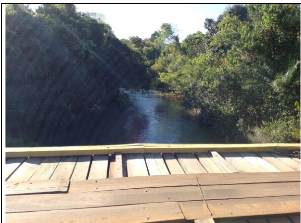
Visto lado Jusante da ponte de madeira sobre o Rio Jangada
